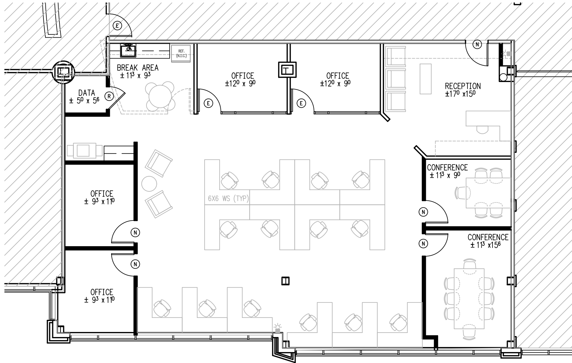
PLAN SCALE: 1/8" = 1'-0"
